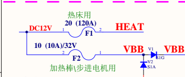
温度保险丝
