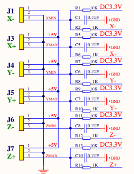
限位开关
